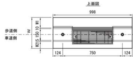
寸法表(mm)
