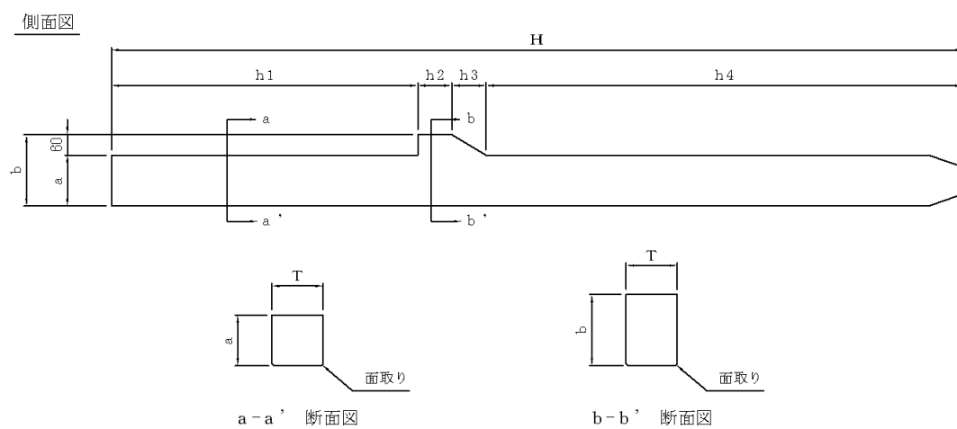
寸法・重量表（12×12）
