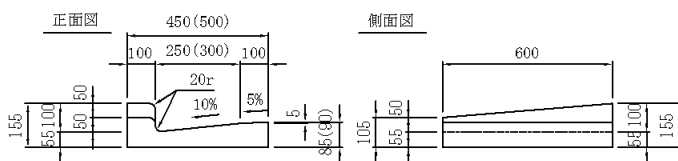
切下げ左 (H=50-100) 250B(300)
