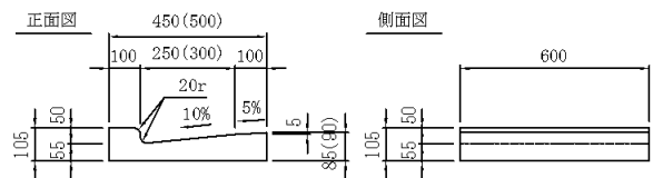
出入口用 (H=50) 250B(300)
