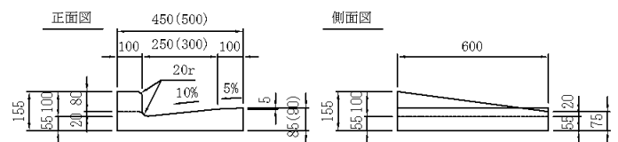
切下げ右 (H=20-100) 250B(300)
