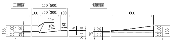
切下げ左 (H=20-100) 250B(300)
