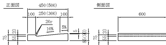
出入口用 (H=20) 250B(300)
