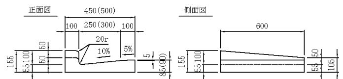
切下げ右 (H=50-100) 250B(300)
