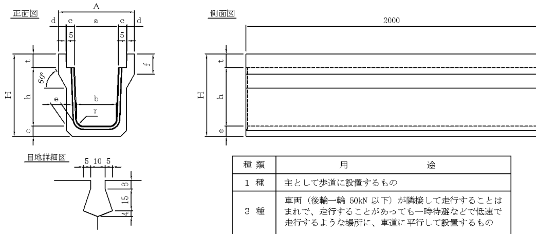
寸法表 (1 種)
