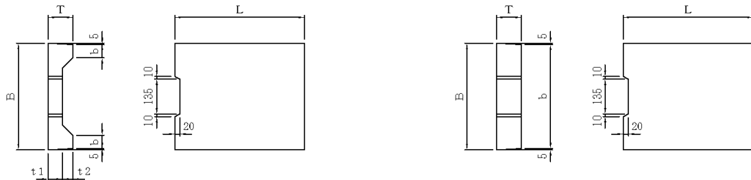
寸法表 (1 種)
