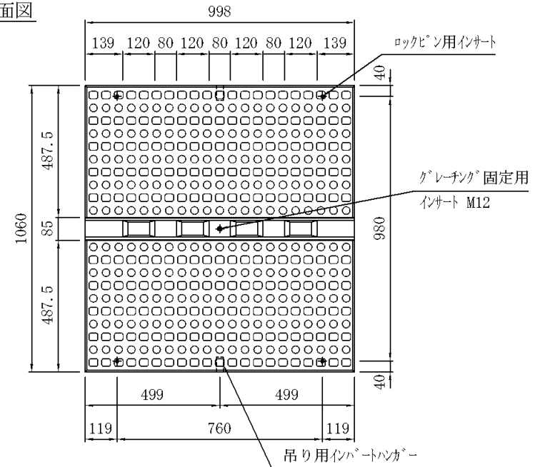
平面図
