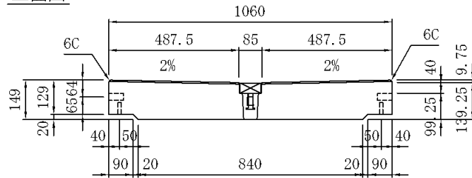
正面図
