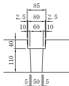
詳細寸法図
