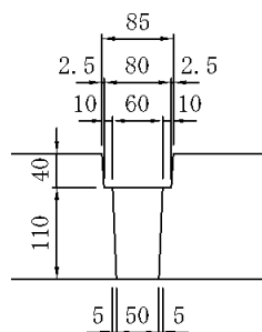
詳細寸法図
