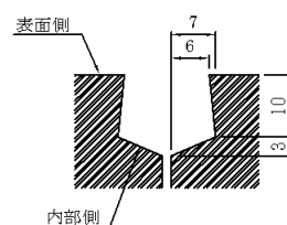
目地詳細図
