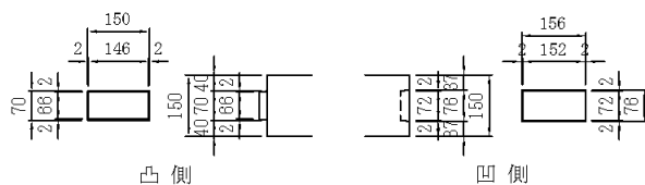
継手詳細図
