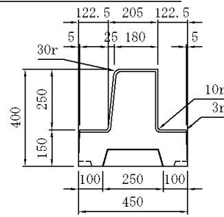
目地詳細図
