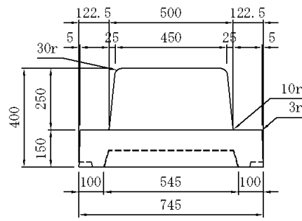
目地詳細図
