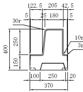
目地詳細図
