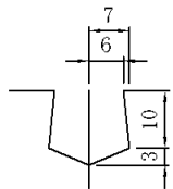
目地詳細図
