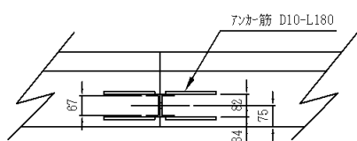
ジョイント部詳細図
