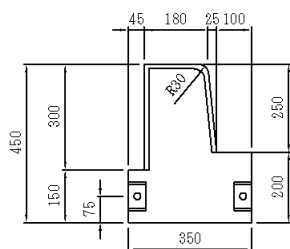
I 型 W=560kg
