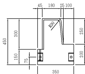
II 型 W=560kg
