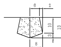
目地部詳細図
