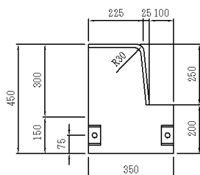
III 型 W=624kg
