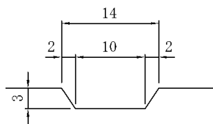
シー目地詳細図
