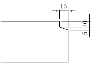
目地詳細図
