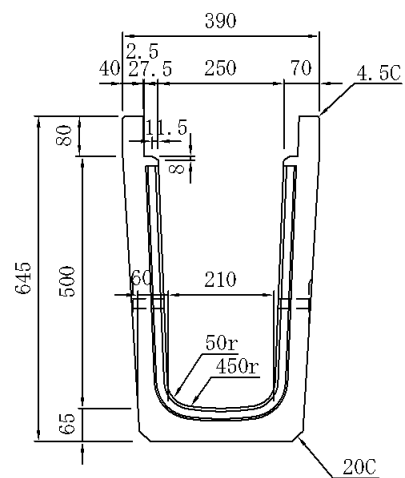
構造図
