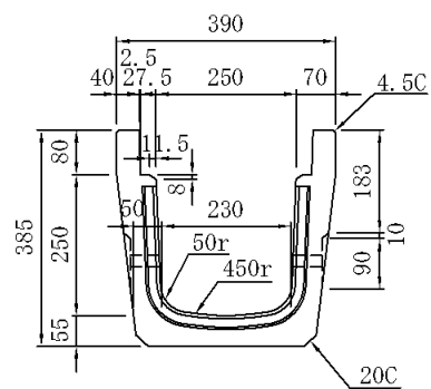
構造図
