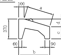
平面図
