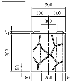
平面図
