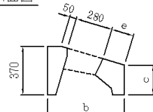
B断面図
