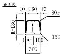
端部目地詳細図
