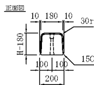
端部目地詳細図
