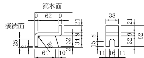
フランジ詳細図
