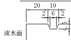
本体目地詳細図
