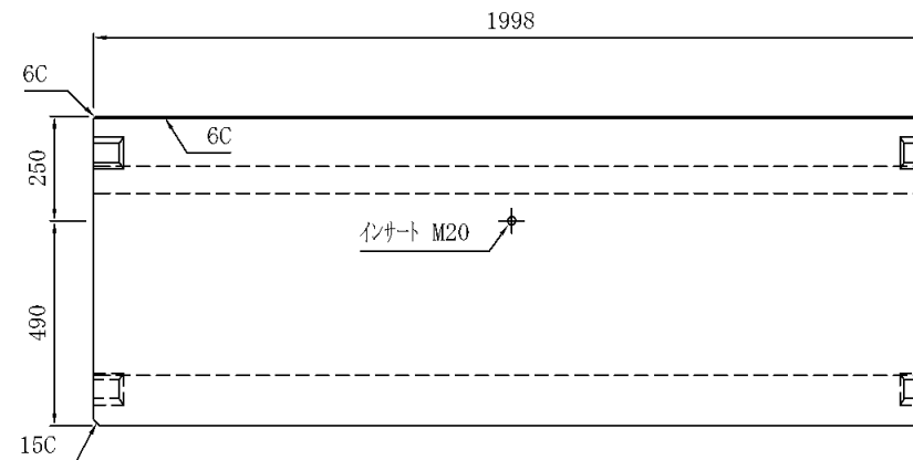
側面図
