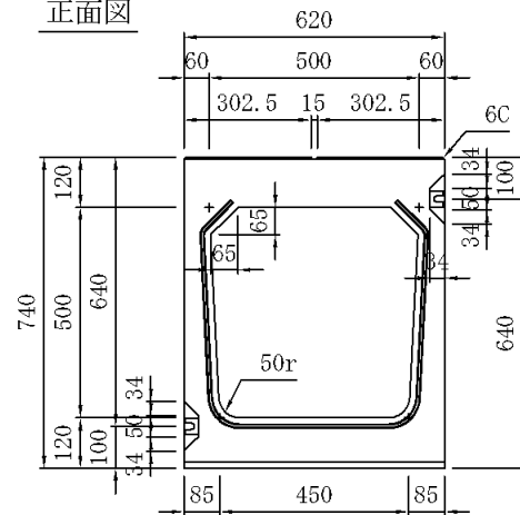
正面図
