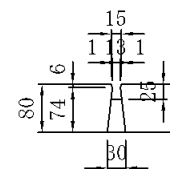
スリット部詳細図
