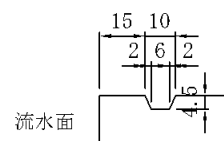
本体目地詳細図
