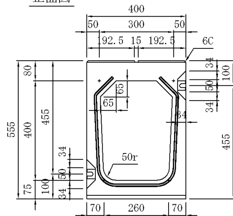
正面図
