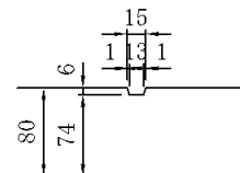
天端詳細図
