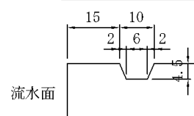
本体目地詳細図
