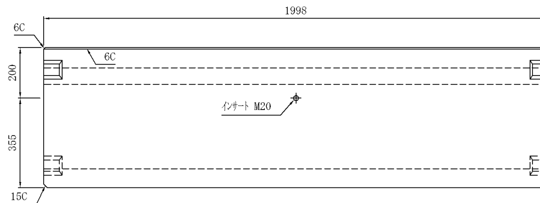
側面図
