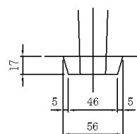
歩車道下部詳細図
