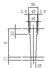
ボルト穴詳細図
