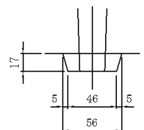
歩車道下部詳細図
