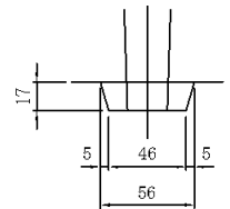
歩車道下部詳細図
