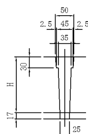
ボルト穴詳細図
